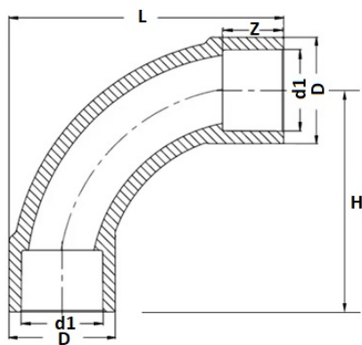
Отвод плавный клеевой 90° ПВХ IPS d50
