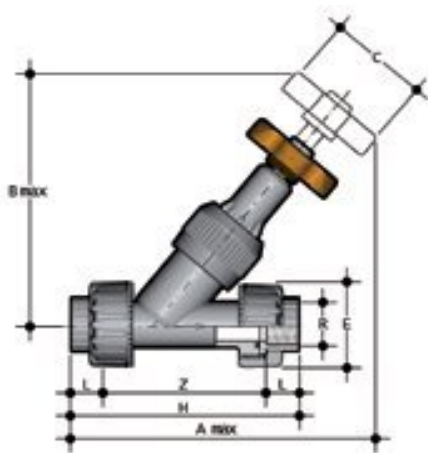
Угловой вентиль VVUFV ПВХ с резьбовыми окончаниями, EPDM, FIP R1" (DN25)
