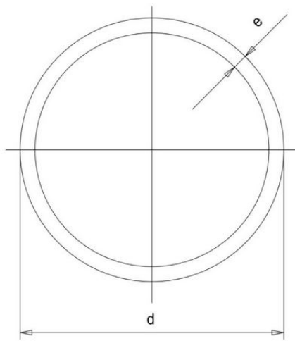
Напорная труба PP-H Simona, PN2.5 d63
