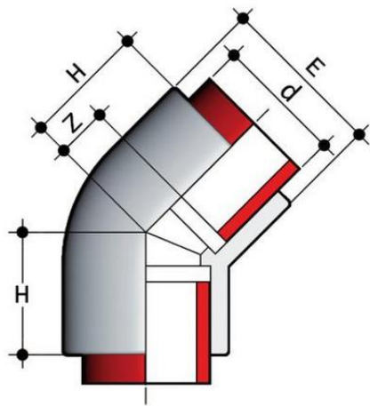
Отвод ПВДФ 45° d32 SDR21 PN16
