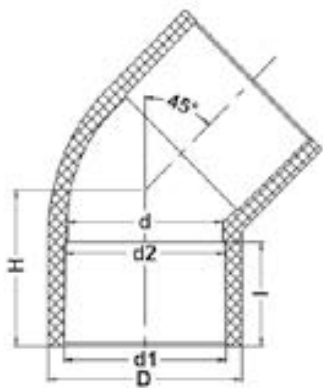
Отвод 45° ХПВХ IPS (Model A) d110 PN16
