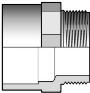
Двойной муфтовый адаптер с НР ПВХ FIP 90x75x3
