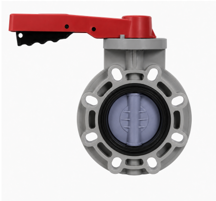
Затвор дисковый в корпусе FRPP (диск - ХПВХ) с рукояткой промышленного применения FKM IPS d110 (DN90)
