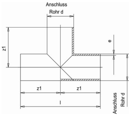
Тройник ПВДΦ 90° (Simona) d110 SDR33 PN10
