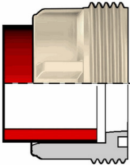
Муфтовая вставка ПВДФ d50 SDR21 PN16
