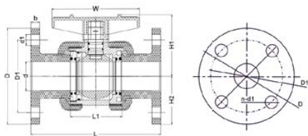
Шаровой кран IVKD ПВДФ с фланцевыми окончаниями (FKM) d90 (DN80)
