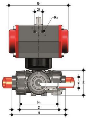
3-х ходовой шаровой кран ТКД с пневмоприводом с муфтовыми окончаниями, L-шар (уплотнение EPDM) PP-H d32 (DN25)
