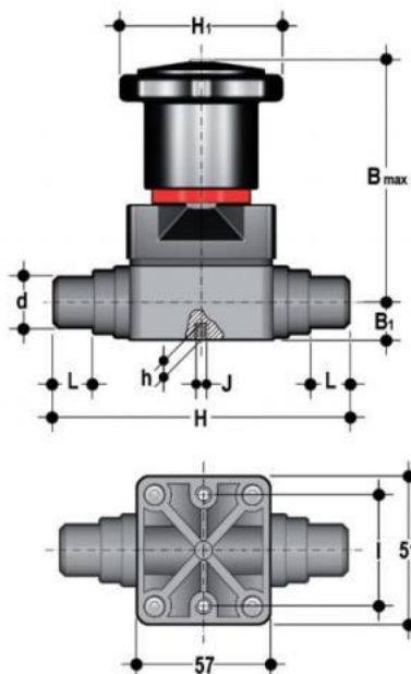
Компактный мембранный клапан PBX с пневмоприводом, CM, EPDM, FIP d20 (DN15)
