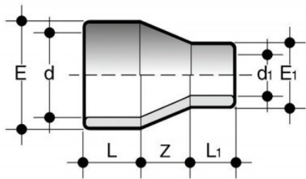
Муфта редукционная ПВХ FIP 400x315
