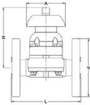
Мембранный клапан IDK ПВХ с фланцевыми окончаниями, EPDM, IPS d90 (DN80)
