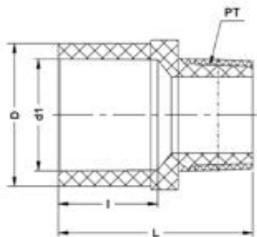
Муфта с НР ХПВХ IPS 40x1¼" PN16
