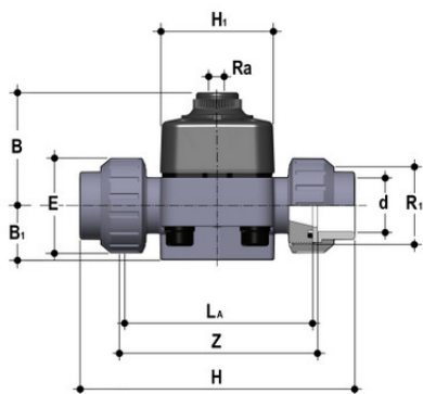
Мембранный клапан ПВХ с пневмоприводом прямого действия, DK, EPDM, FIP d50 (DN40)
