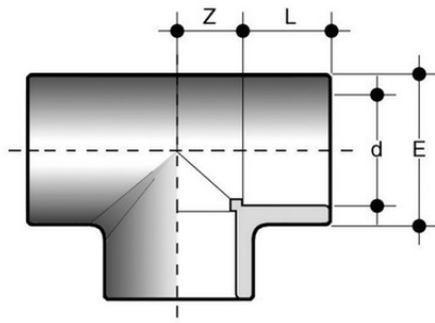
Тройник равнопроходной клеевой 90° ПВХ FIP d110
