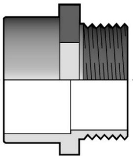
Адаптер с наружной резьбой PP-H FIP 40x1 1/4 SDR11 PN10
