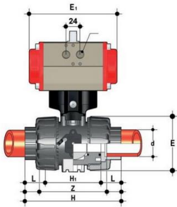
Шаровой кран VKD с пневмоприводом НО с муфтовыми окончаниями (уплотнение FKM) PP-H d40 (DN32)
