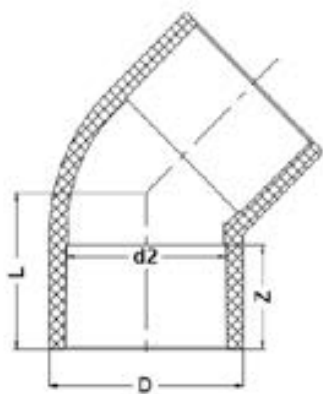
Отвод 45° ХПВХ IPS (Model B) d400 PN10
