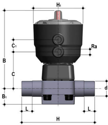
Мембранный клапан ДК ХПВХ с пневмоприводом НО, PN10, втулочные окончания d40 (DN32)
