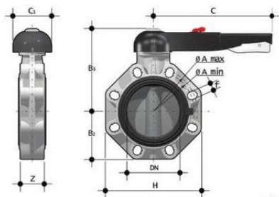
Дисковый затвор FK ХПВХ с рукояткой d75 (DN65)
