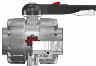
Шаровой кран промышленного применения VKD ХПВХ с резьбовыми окончаниями, DN65-100 R2 1/2" (DN65)
