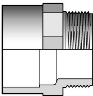
Двойной муфтовый адаптер с НР ПВХ FIP 20x16x3/8
