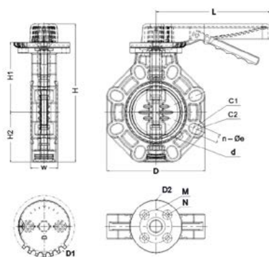
Затвор дисковый ХПВХ с рукояткой EPDM IPS d63 (DN50)
