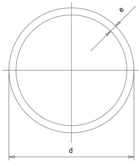
Труба ПВДФ (Simona) d180 SDR33 PN10
