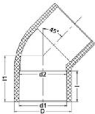
Отвод для растровной сварки ПВДФ 45° d110 PN 16
