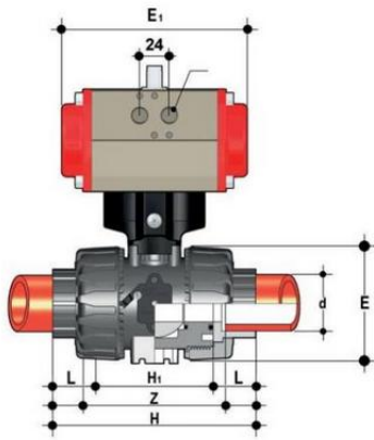
Шаровой кран VKD с пневмоприводом ДвД с муфтовыми окончаниями (уплотнение EPDM) PP-H d50 (DN40)
