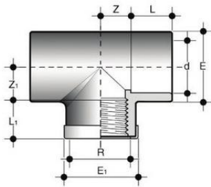
Тройник переходной ВР с усиливающим кольцом ХПВХ 32x1" PN16
