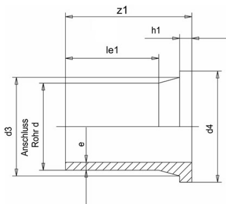
Бурт PP-H Simona d140 SDR11 PN6
