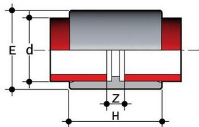
Муфта соединительная PP-H FIP PN10
