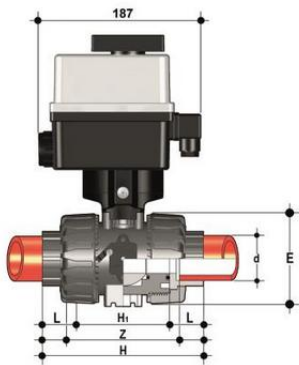
Шаровой кран VKD с эл.приводом 90-240V, муфтовые окончания (уплотнение EPDM) PP-H d32 (DN25)
