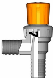
Мембранный кран RMRV ПВХ, резьбовое соединение, EPDM, FIP d15 (DN15)
