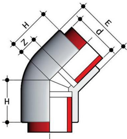
Отвод 45° для раструбной сварки PP-H FIP PN10
