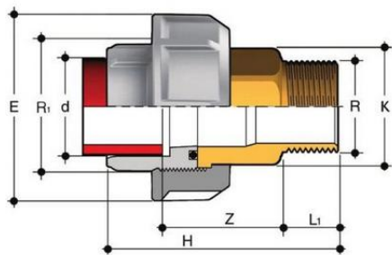
Муфта разборная переходная РР-Н / латунь, НР (EPDM) FIP 50x1 1/2 PN10
