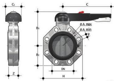
Дисковый затвор промышленного применения FKOMLM с рукояткой (уплотнение EPDM) PP-H d200 (DN200)
