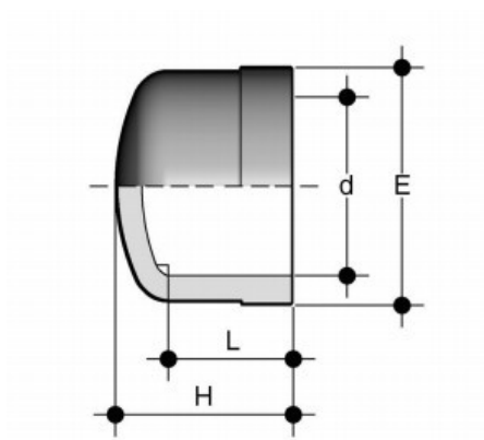
Заглушка ХПВХ d32 PN16
