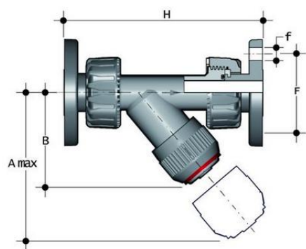
Грязевой фильтр RV ХПВХ с фланцевыми окончаниями d25 (DN20)
