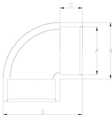
Отвод клеевой 90° ПВХ Hidroten d50
