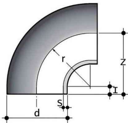
Отвод 90° для стыковой сварки PP-H FIP d450 SDR11 PN6
