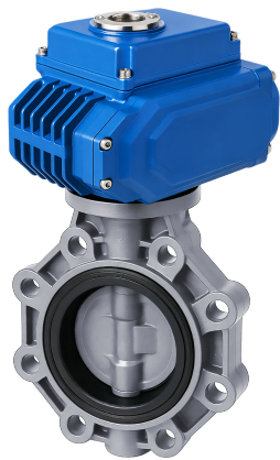
Дисковый затвор IFK ХПВХ с электрическим приводом 24V DC, FKM, IPS d110 (DN90)
