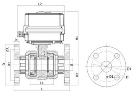
Шаровой кран IVKD ПП-гомополимер с эл.приводом 220V AC, фланцевые окончания, FKM, IPS d25 (DN20)
