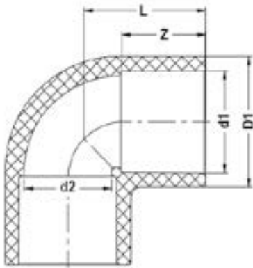
Отвод ПВДФ 90° (IPS) d110 PN 16
