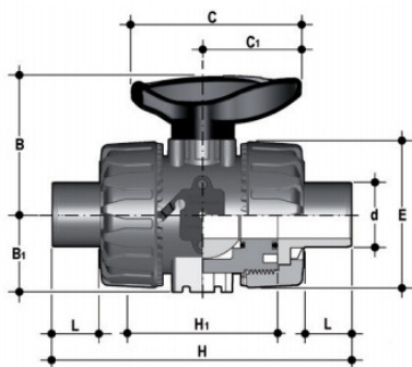
Шаровой кран ПВХ промышленного применения VKD со втулочными окончаниями, FKM, FIP d16 (DN10)
