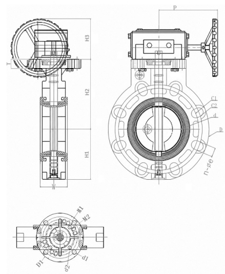
Затвор дисковый в корпусе FRPP (диск - ПВДФ) с редуктором промышленного применения FKM IPS d225 (DN200)
