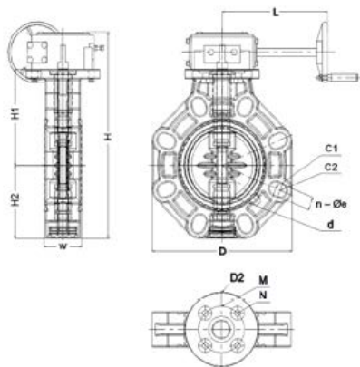
Затвор дисковый ПБХ с редуктором промышленный IPS (Model A) d12" (DN300)
