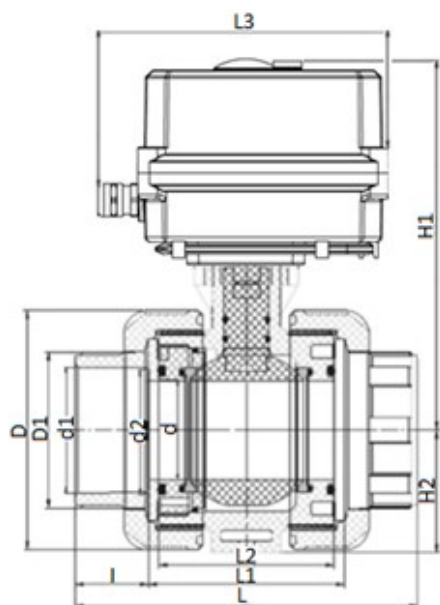
Шаровой кран IVKD ПВДФ с эл.приводом 24V DC, муфтовые окончания, EPDM, IPS d75 (DN65)
