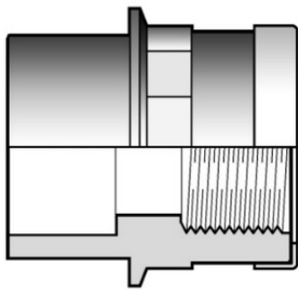
Двойной муфтовый адаптер с ВР и усиливающим кольцом ПВХ FIP 25x20x1/2
