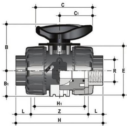
Шаровой кран для регулирования потока VKRFM с резьбовыми окончаниями (уплотнение FKM) PP-H R1¼" (DN32)
