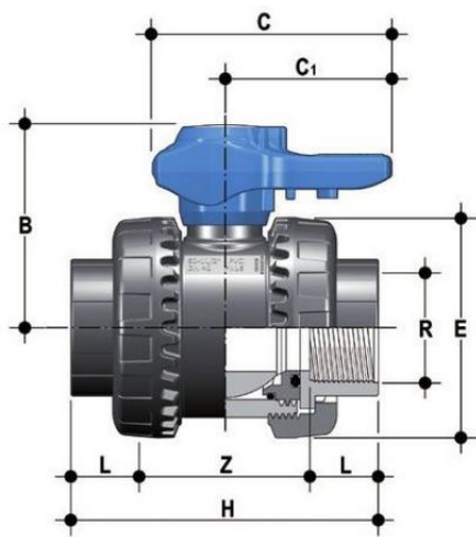
Шаровой кран ПВХ общего применения VEE; муфтовые окончания с ВР, EPDM, FIP R1" (DN25)
